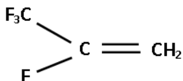
Figure 4.1 Structure du R-1234yf
