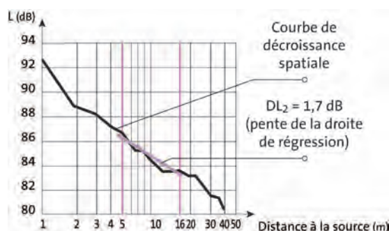
Exemple de courbe de décroissance et de calcul de DL_2
